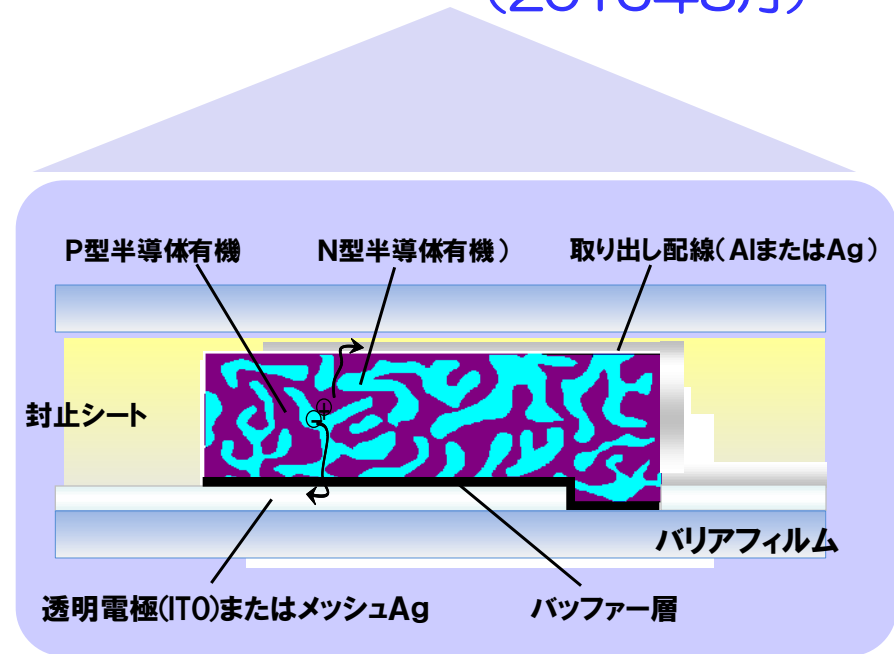
OPVの発電部断面イメージ バルクヘテロ構造
